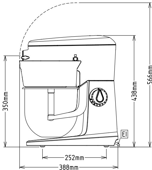
Zij aanzicht
